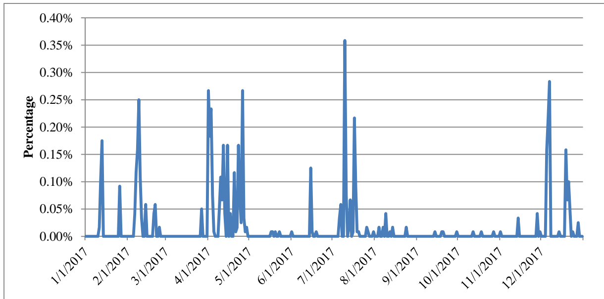
Figure N.1 – Daily LOLP
